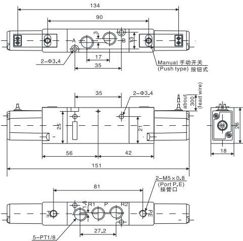
TVZ5 3 / 5 20-□G
