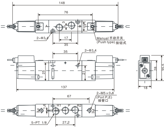
TVZ5 3 / 5 20-□L/LZ
