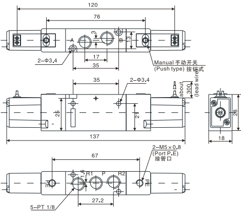
TVZ5 3 / 5 20-□G
