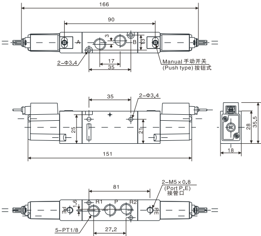
TVZ5 3 / 5 20-□L/LZ
